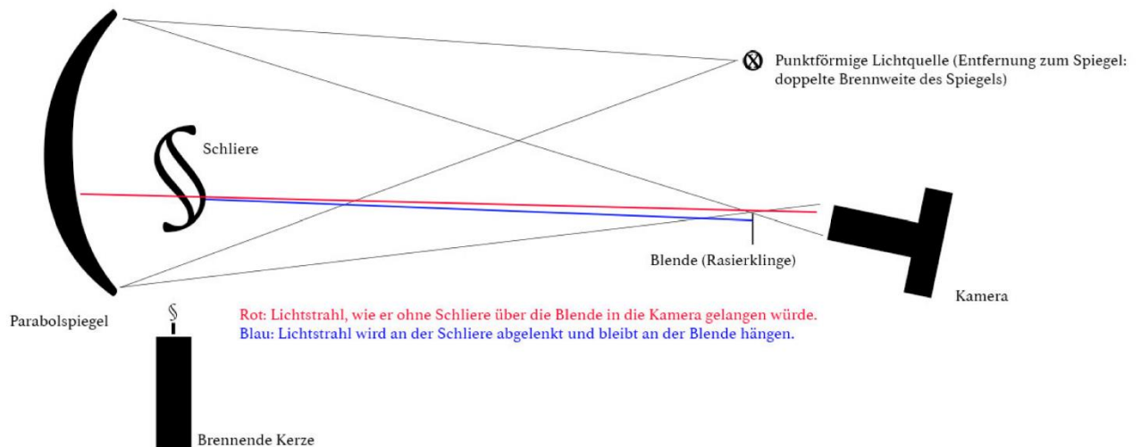
Abb. 1: Ein Prinzip des Aufbaues wie er in den Versuchen verwendet wurde /2/.
