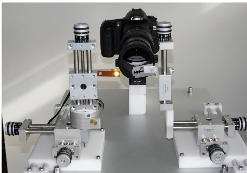
Abb. 2: Feinjustiereinheit sowohl für die LED als auch der Rasierklinge in allen Dimensionen. Rasierklinge und LED sind dann im identischen Abstand zum Spiegel – 2 mal Brennweite des Spiegels.
