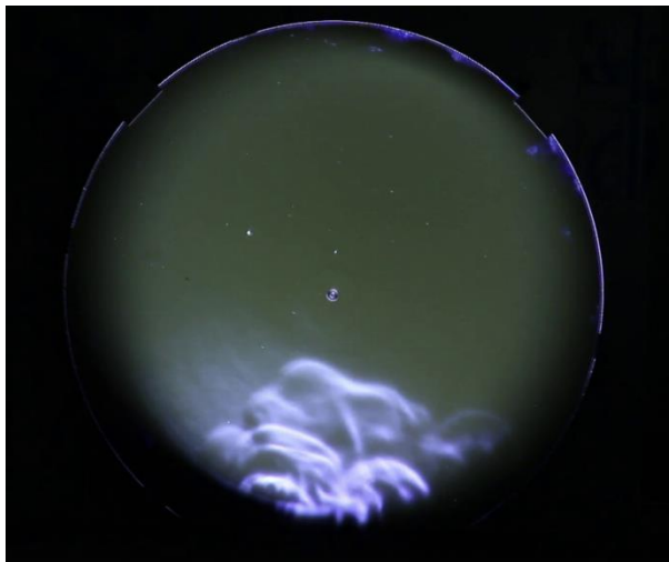
Abb. 7: entstehende Konvektionsströmung über einer aufgeheizten Platte von ca. 60 °C. Die Konvektionsströmung wird durch die Anströmung von oben mit einer FFU unterdrückt.
