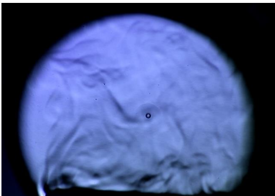
Abb. 8: Freie Konvektion über der aufgeheizten Platte
