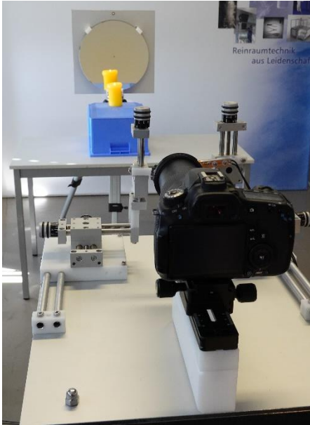
Abb. 3: Darstellung des Gesamtaufbaus aus Blickrichtung der Kamera hin zum Spiegel. Die Kamera ist auf dem horizontalen Schlitten verfahrbar.
